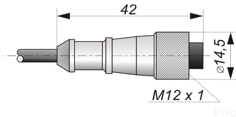
Габаритный чертеж
