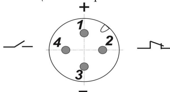
Цоколевка разъема
